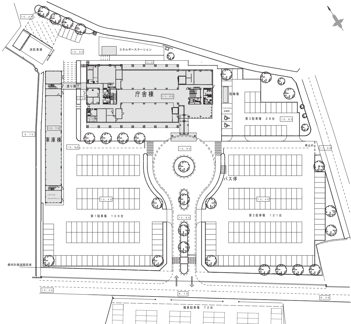
【防災センター兼揖斐川町庁舎土地利用計画図】
