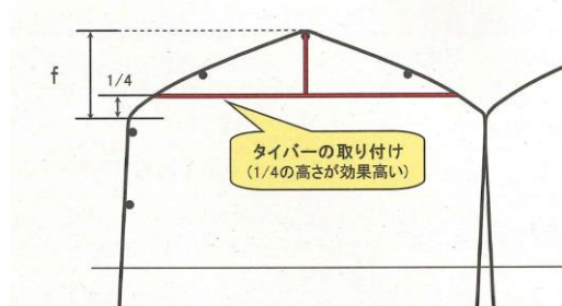
タイバーによる肩部の補強事例
